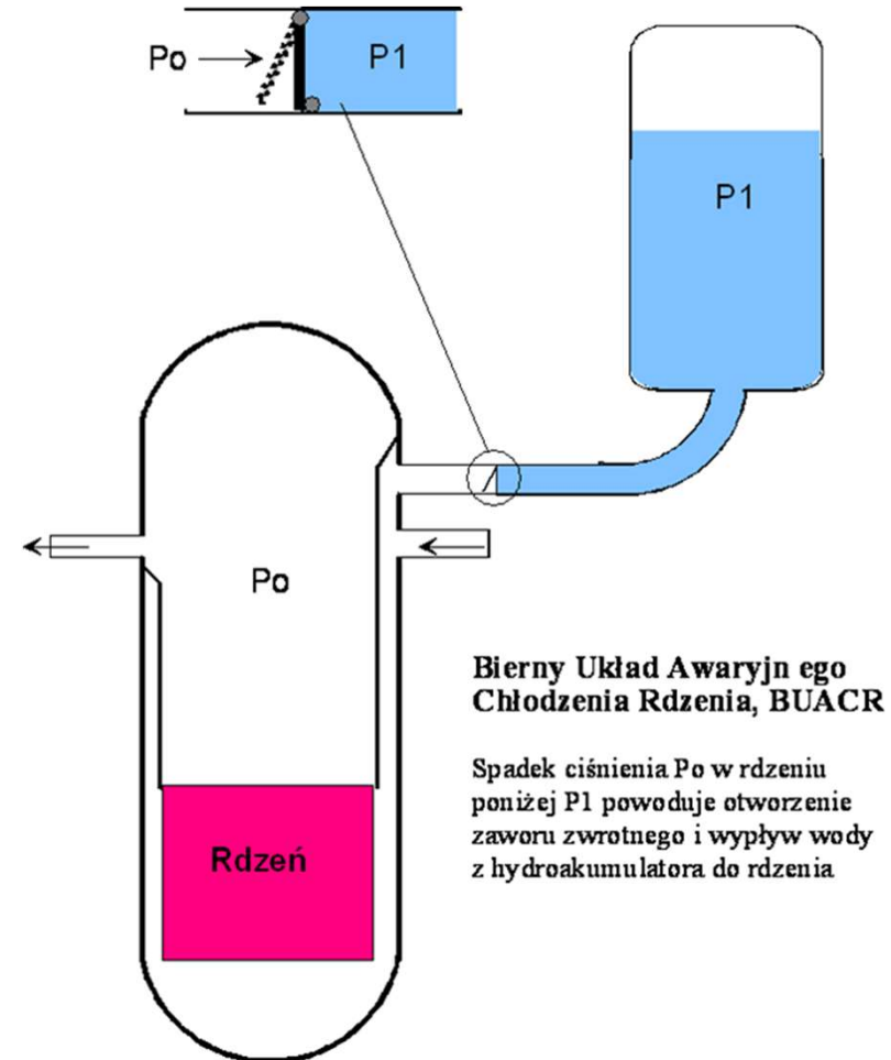
Wykorzystanie energii sprężonego gazu (azot) i zastosowanie klap zwrotnych w BUACR
