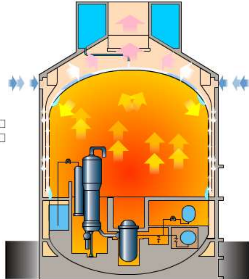
Wykorzystanie grawitacji, konwekcji naturalnej i parowania / skraplania - pasywne chłodzenie obudowy bezpieczeństwa reaktora AP1000
