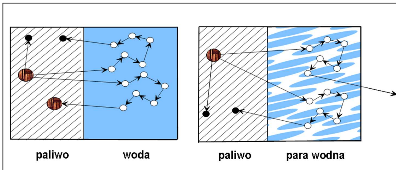
Ilustracja bilansu neutronów (wychwyt, spowalnianie, ucieczka) w reaktorze wodnym przed i po odparowaniu wody
