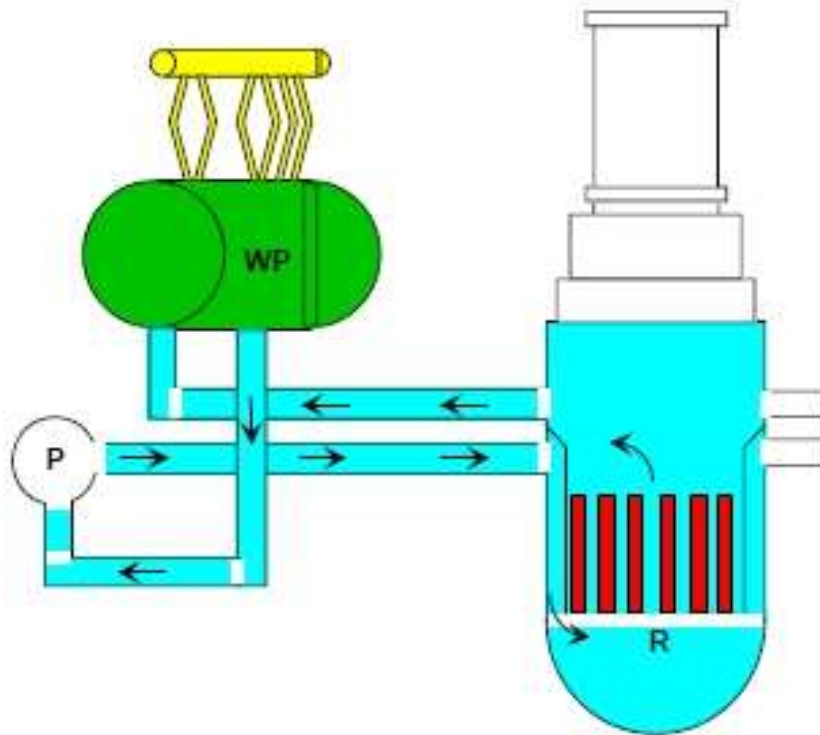
Wykorzystanie konwekcji naturalnej w układzie chłodzenia reaktora (WWER) – odbiór ciepła powyłączeniowego
