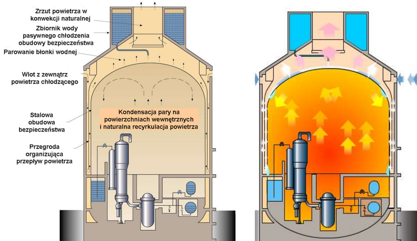
Pasywny układ chłodzenia obudowy bezpieczeństwa AP1000
