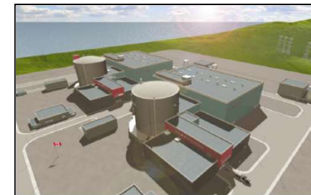
EC6: reaktor ciężkowodny, moc brutto: 750 MWe; SNC Lavalin – Kanada
