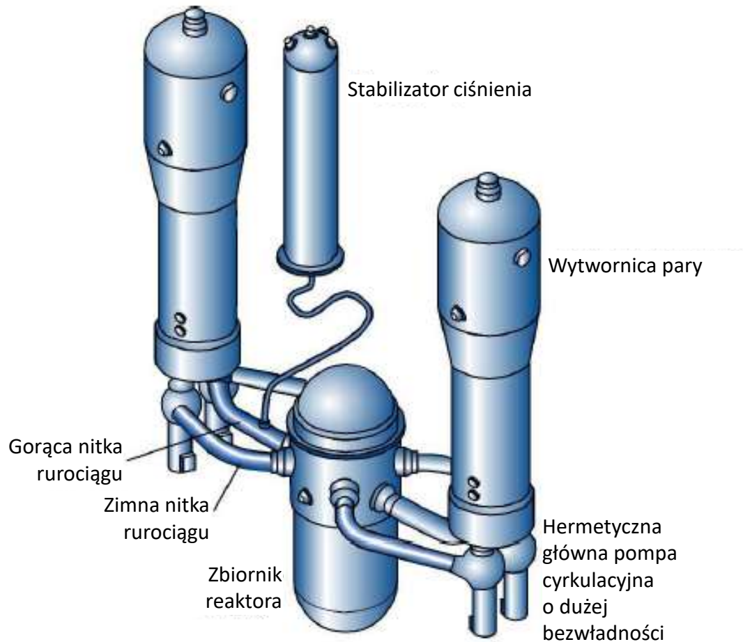
Jądrowy układ wytwarzania pary AP1000
